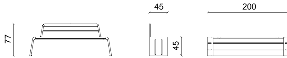
Panchina con schienale Panchina con schienale
