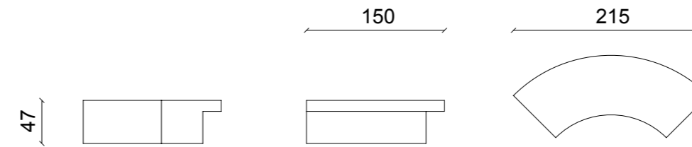
Panchina curva concava Panca curva concava
