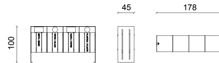
Portarifiuti modulo 4 racc. diff. con cop. Portarifiuti modulo 4 racc. diff. con cop.
