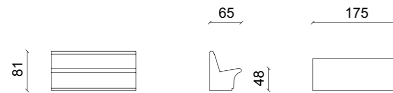
Panca del Golfo modulare dritta Panca del Golfo modulare dritta
