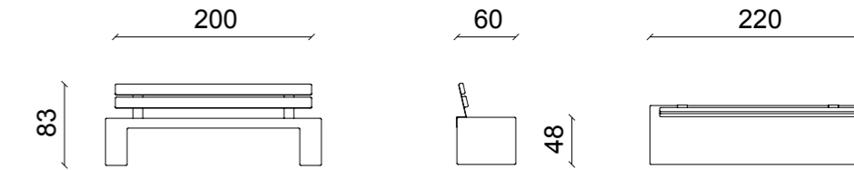
Panca Station con schienale legno Panca Station con schienale legno
