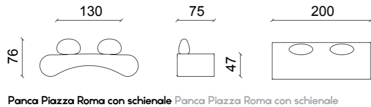
Panca Piazza Roma con schienale Panca Piazza Roma con schienale
