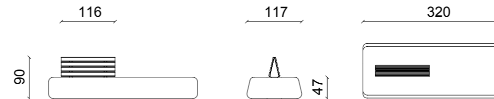
Panchina Dialogo Maxi con schienale corto Panchina Dialogo 320 con schienale corto in legno
