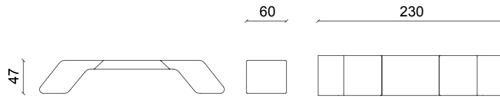
Panchina Mix con piano con parte in legno doppia Panchina Mix
