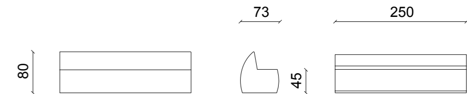
Panca MD con schienale
