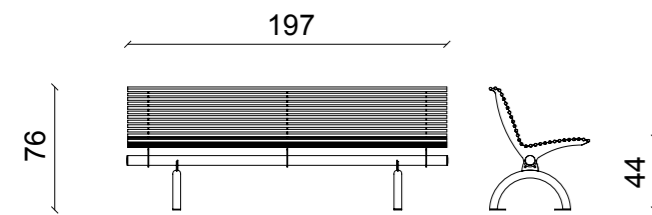
Panchina con schienale Panchina con schienale
