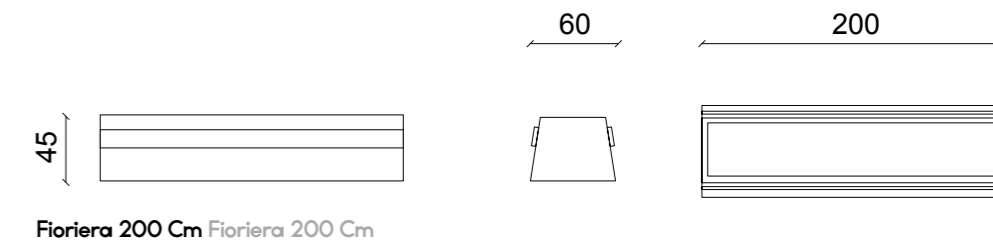
Fioriera 200 Cm Fioriera 200 Cm
