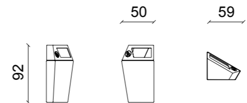
Portarifiuti Block Portarifiuti Block
