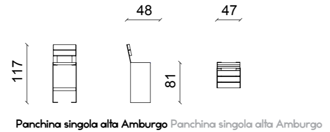
Panchina singola alta Amburgo Panchina singola alta Amburgo
