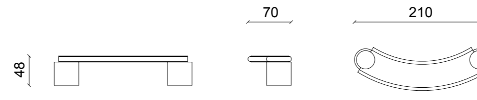
Panchina curva modulare Panca curva modulare
