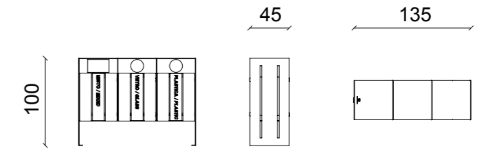
Portarifiuti modulo 3 racc. diff. senza cop. Portarifiuti modulo 3 racc. diff. senza cop.
