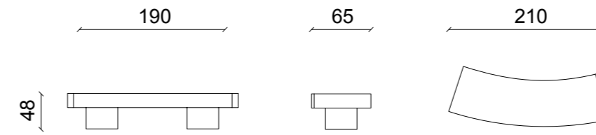
Panca Onda corta piana Panca Onda corta piana
