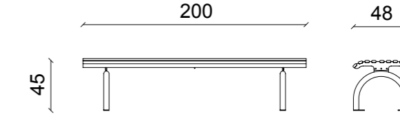
Panchina piana Panchina piana
