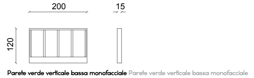
Parete verde verticale bassa monofacciale Parete verde verticale bassa monofacciale
