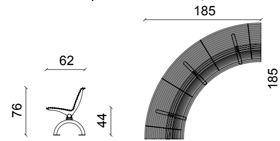
Panchina curva con schienale interno Panchina curva con schienale interno
