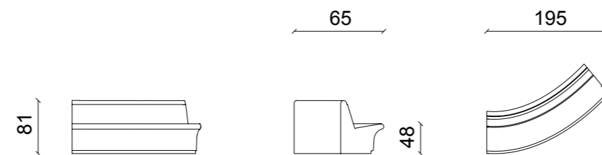
Panca del Golfo modulare convessa Panca del Golfo modulare convessa
