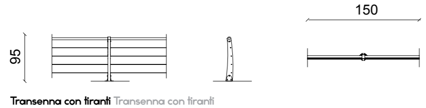
Transenna con tiranti Transenna con tiranti
