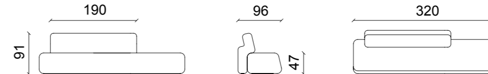
Panchina Dialogo 320 con schienale Panchina Dialogo 320 con schienale
