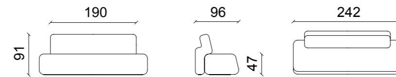
Panchina Dialogo con schienale Panchina Dialogo con schienale
