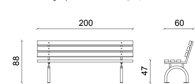
Panchina in legno con schienale Panchina in legno con schienale
